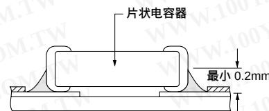
〔回流焊接方式的焊锡用量〕
