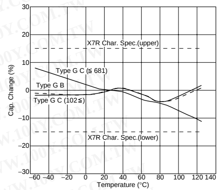
GA3 系列 (GB/GC 型)
