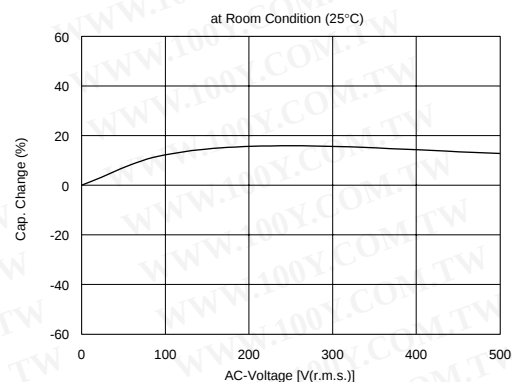
GA3 系列（GD/GF 型，X7R 特性）
