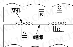
〔靠近 PCB 分离处的芯片安装位置〕
